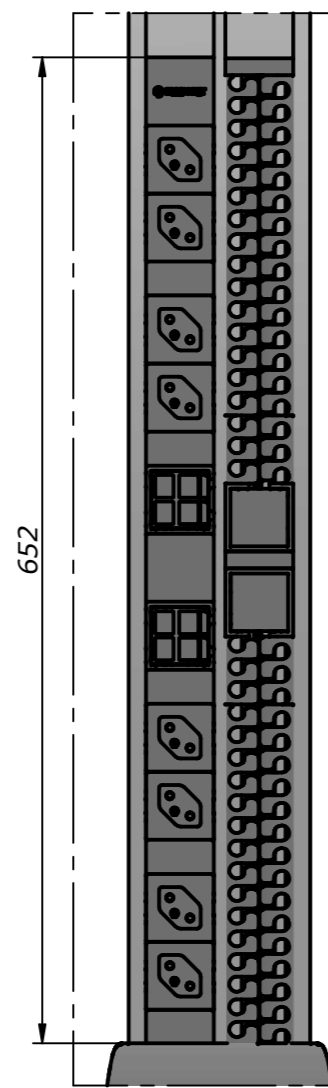
DETALLE A
